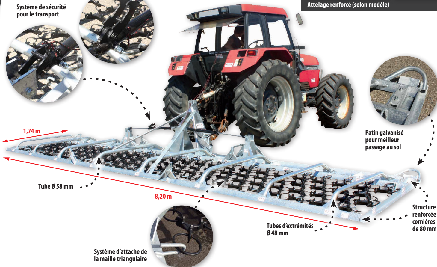
Attelage renforcé (selon modèle)
