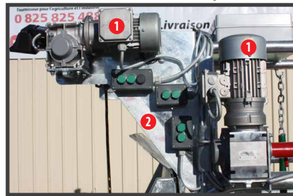
2 Boîtiers de commande du treuil ventral, du lève pattes arrière et des sangles de maintien du bassin
