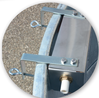
Fixation coffre à flotteur
